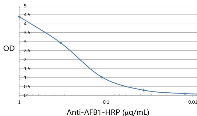
Fig 2. ELISA Titration of anti-AFB1 HRP ( \mu g/mL).
